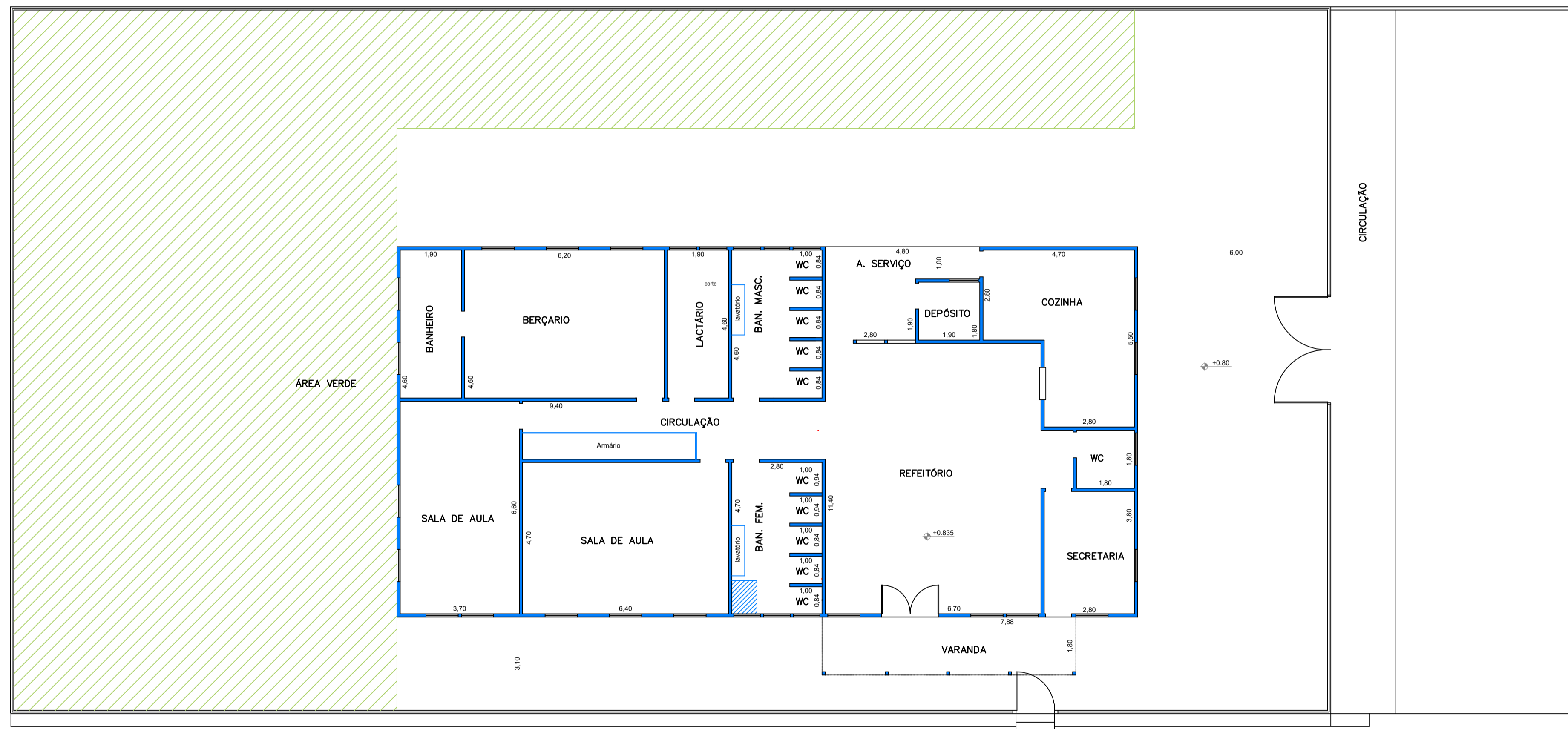
PLANTA BAIXA ESC. 1:100
